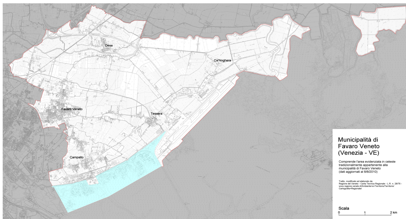
Figura 1. Mappa dell'area considerata e principali località.
